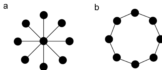
Abb. 2 Betweenness centralities 1 (a) und 0 (b): Schematische Darstellung.
